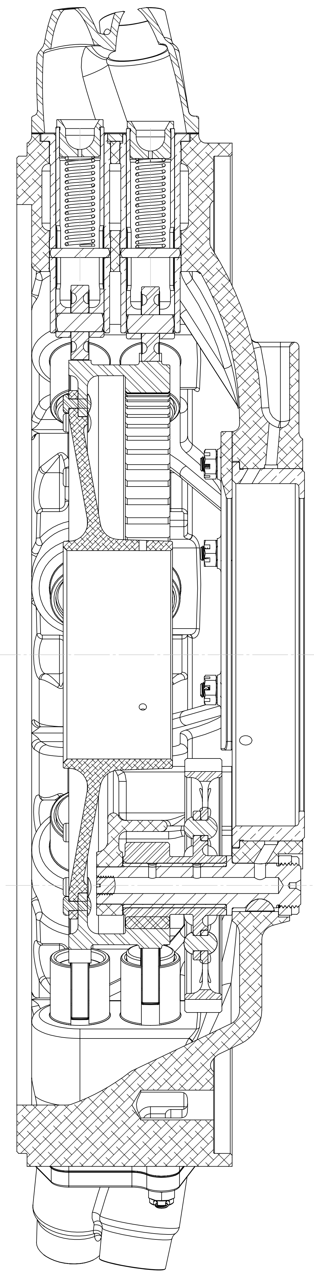
SECTION A-A
