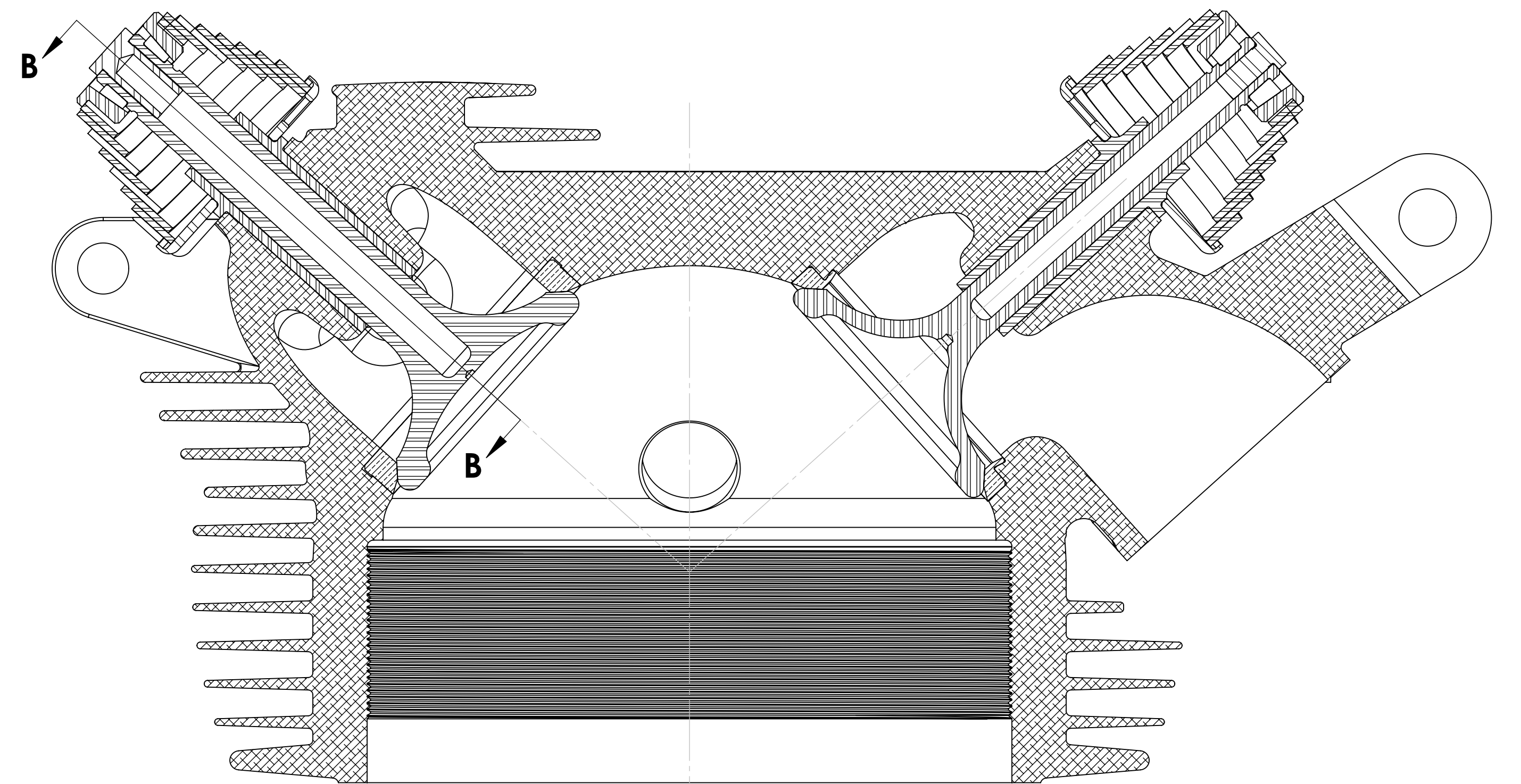
SECTION A-A
