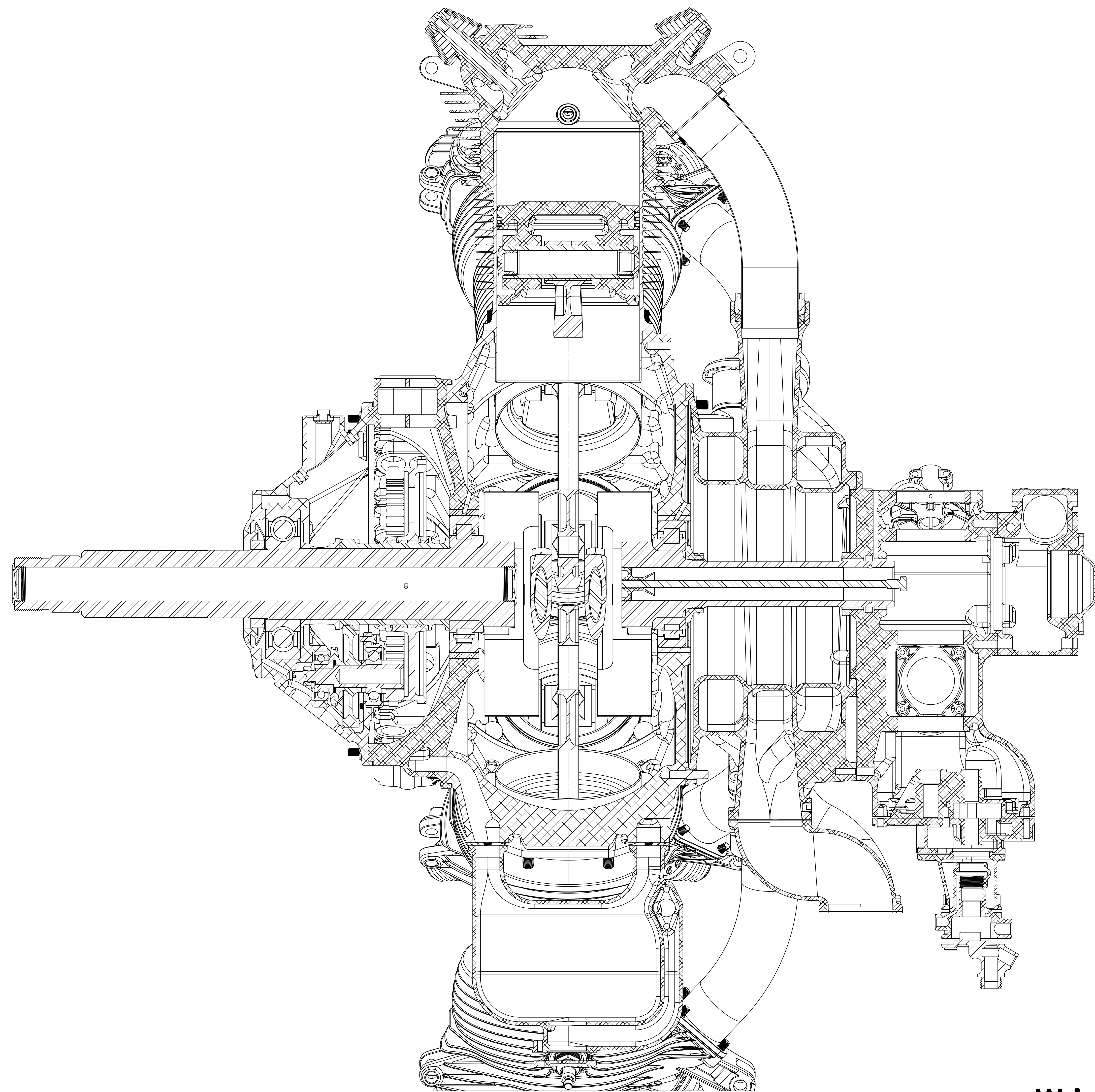
SECTION A-A SCALE 1 : 2
