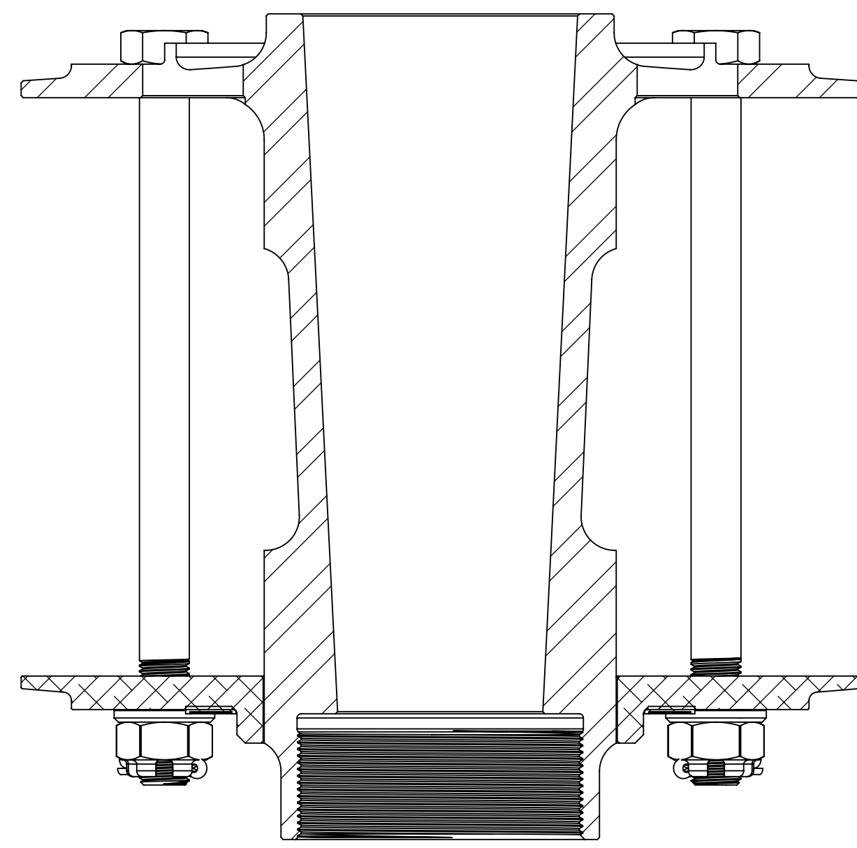
SECTION A-A
